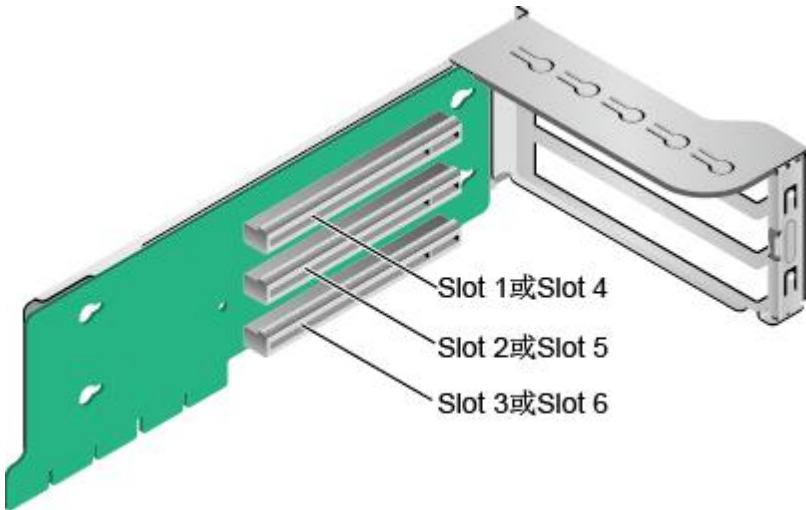
图 5-11 3x8 Riser 卡 1
