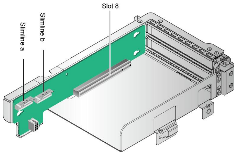
图 5-17 1x16 Riser 卡 7
