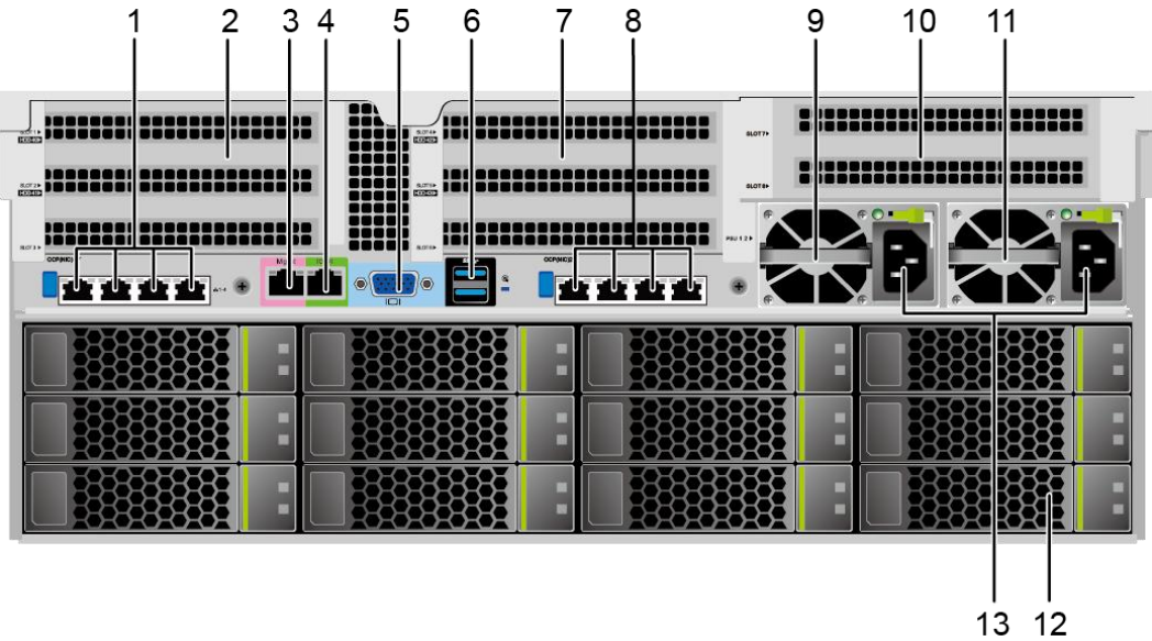
图 5-3 后面板组件
