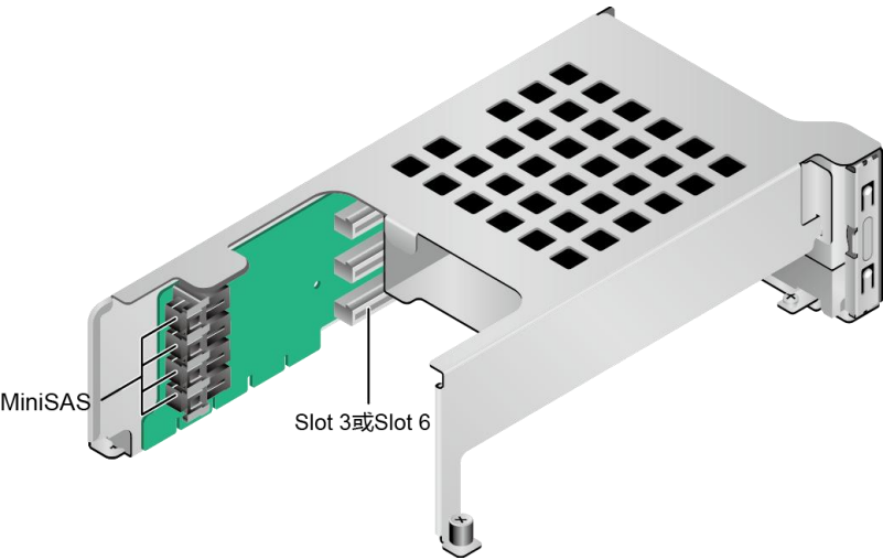
图 5-14 2x2.5 背板 SAS Riser 卡 4
