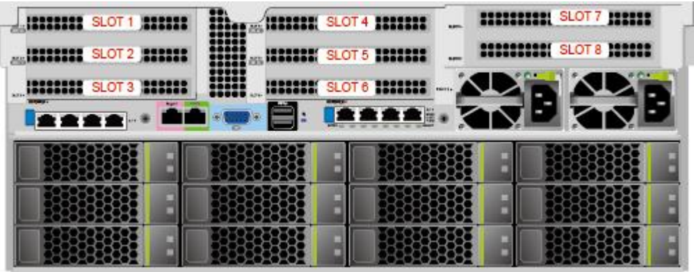
图 5-18 PCIe 插槽
