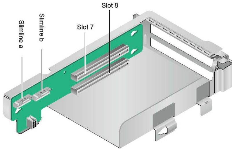
图 5-16 2x8 Riser 卡 6
