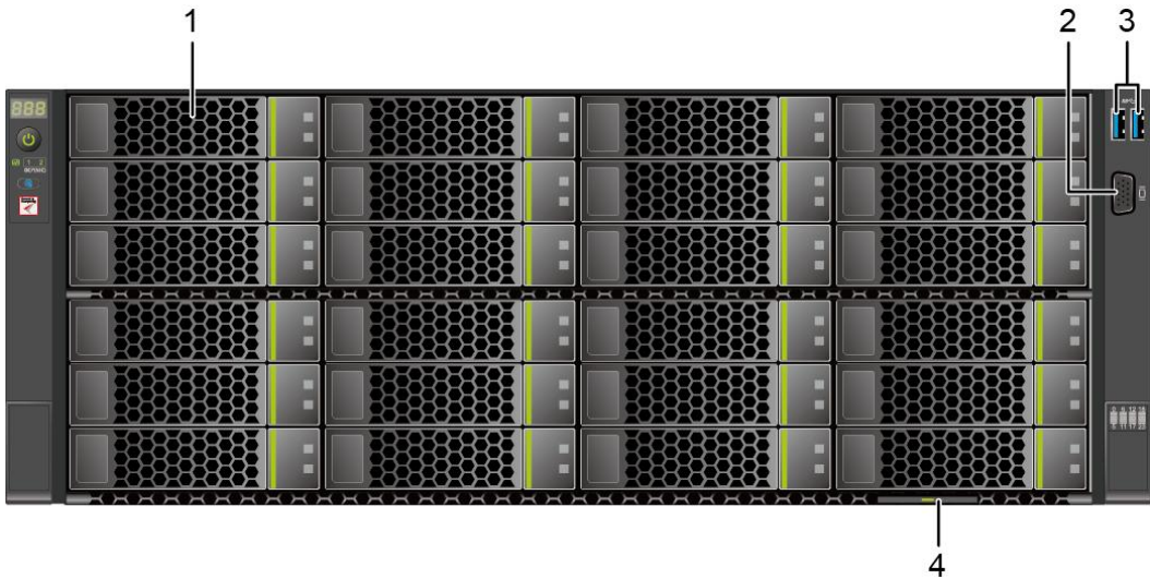
图 5-1 前面板组件
