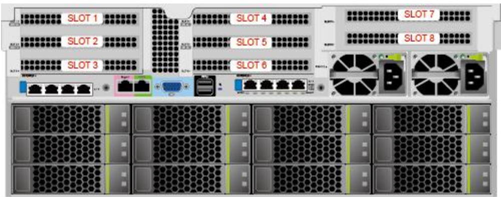
图 4-15 PCIe 插槽
