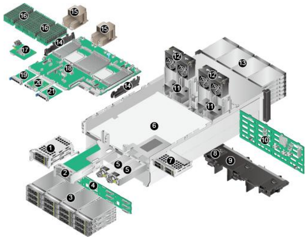
图 4-16 部件
