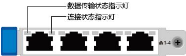
图 4-7 TM210（4xGE 电口）
