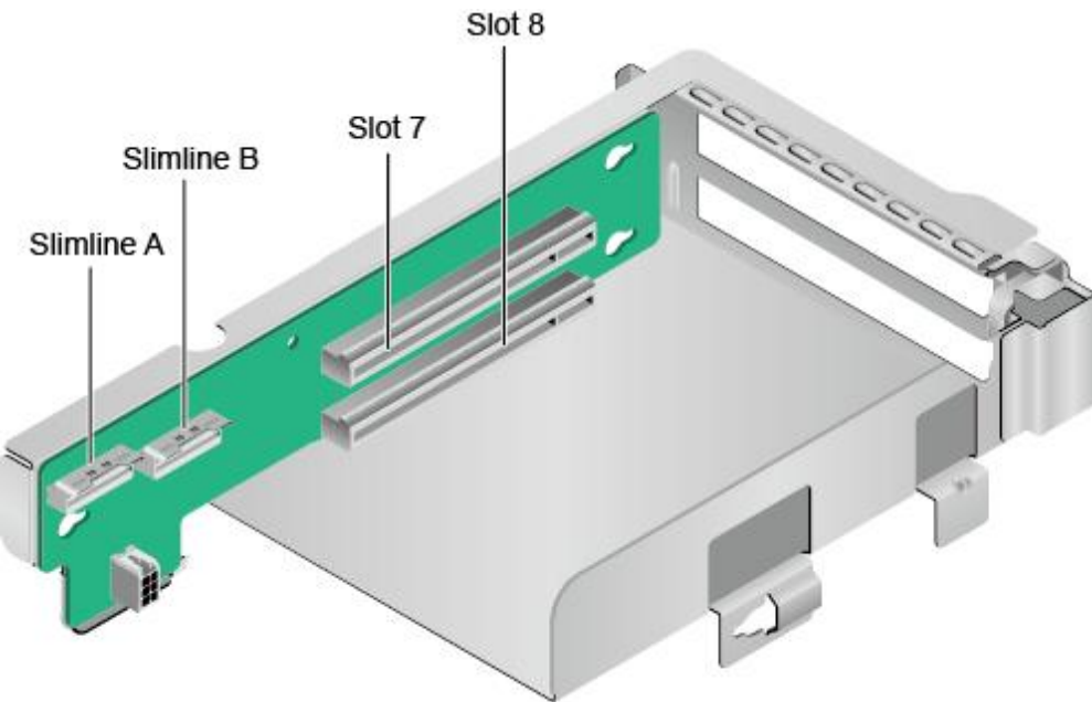
图 4-13 Riser 卡 5（2x8）
