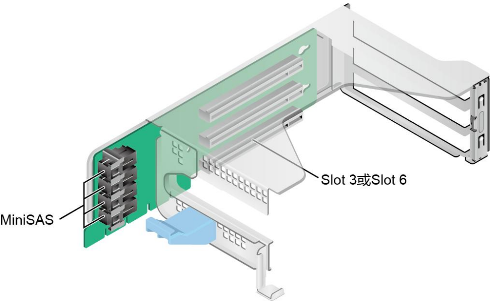
图 4-12 Riser 卡 4（SAS Riser）
