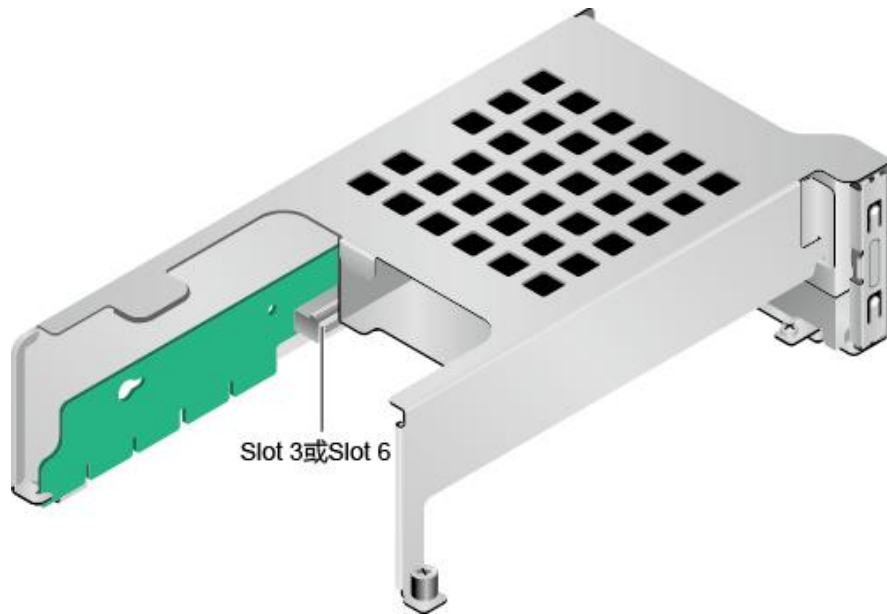
图 4-11 Riser 卡 3（1x16）
