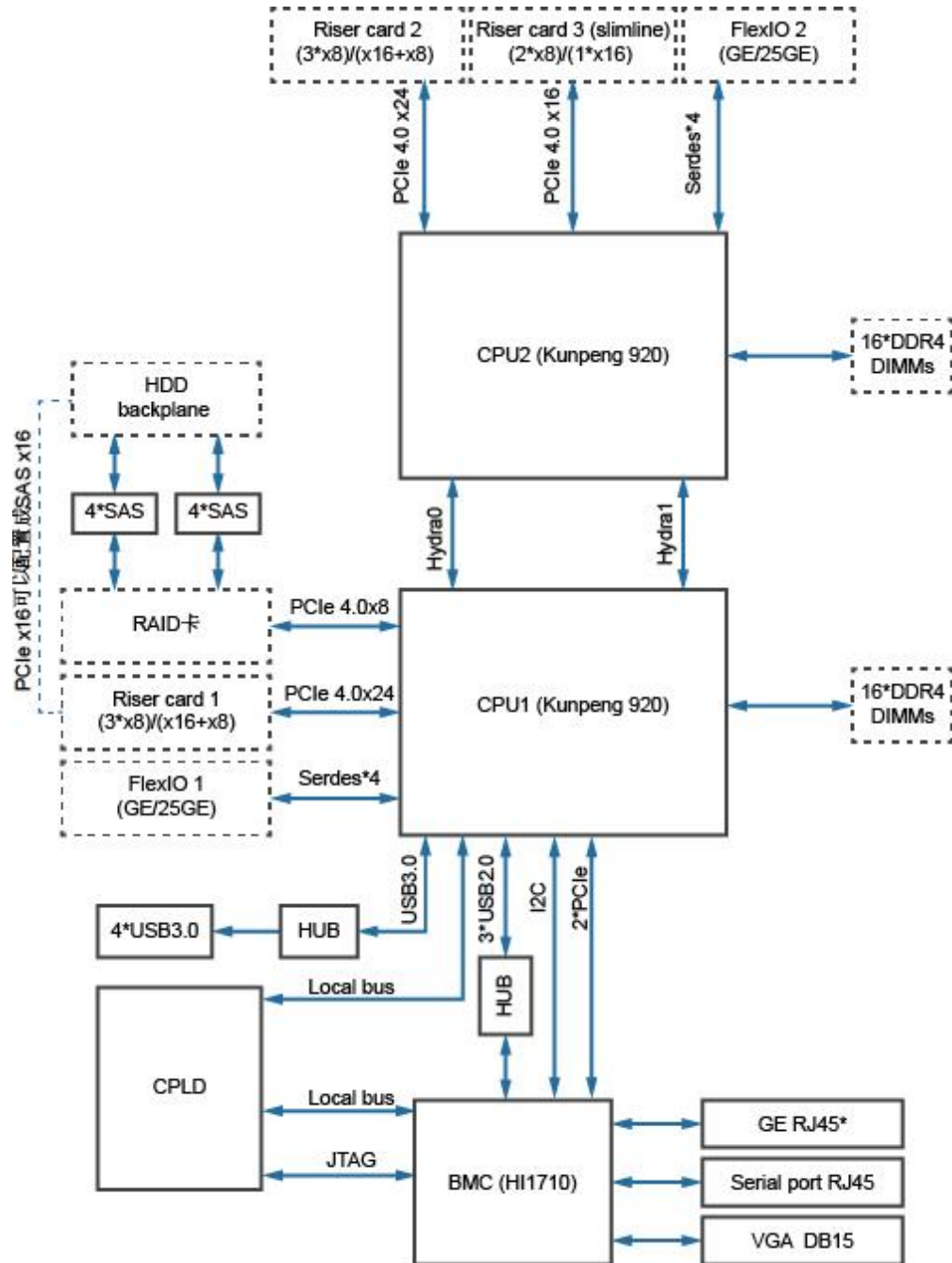
图 3-1 PR410K(4864C)逻辑结构
