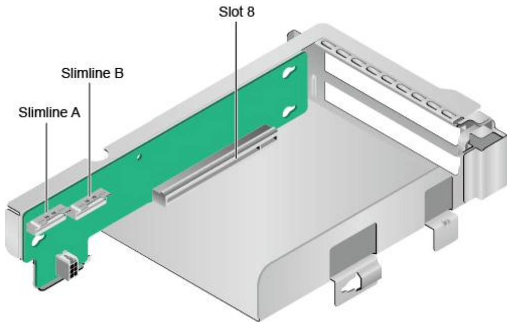
图 4-14 Riser 卡 6 (1x16)
