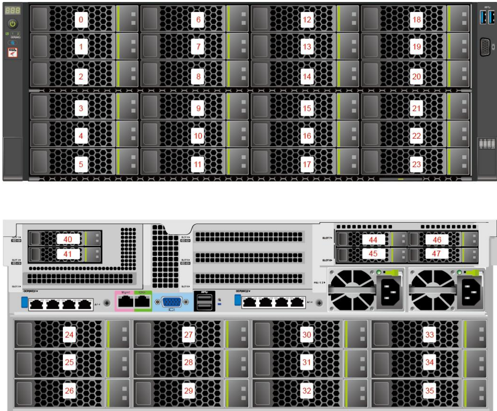
图 6-4 36x3.5 英寸直通/RAID 直通机型的硬盘编号
