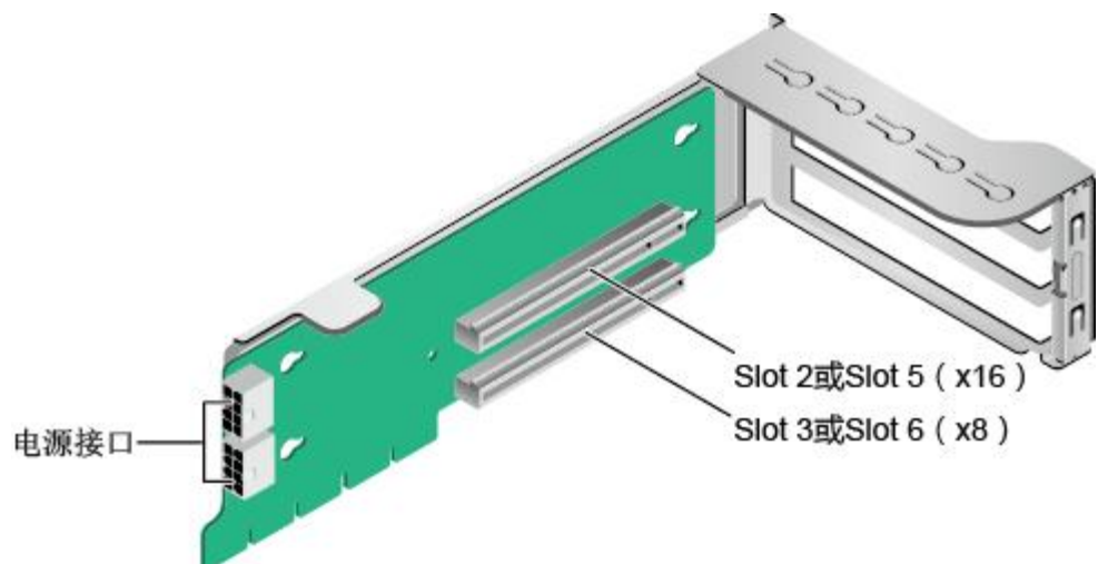
图 4-10 Riser 卡 2 (1x8+1x16)
