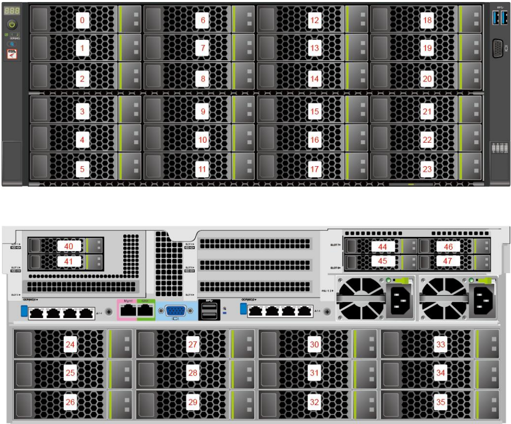
图 6-4 36x3.5 英寸直通/RAID 直机型的硬盘编号
