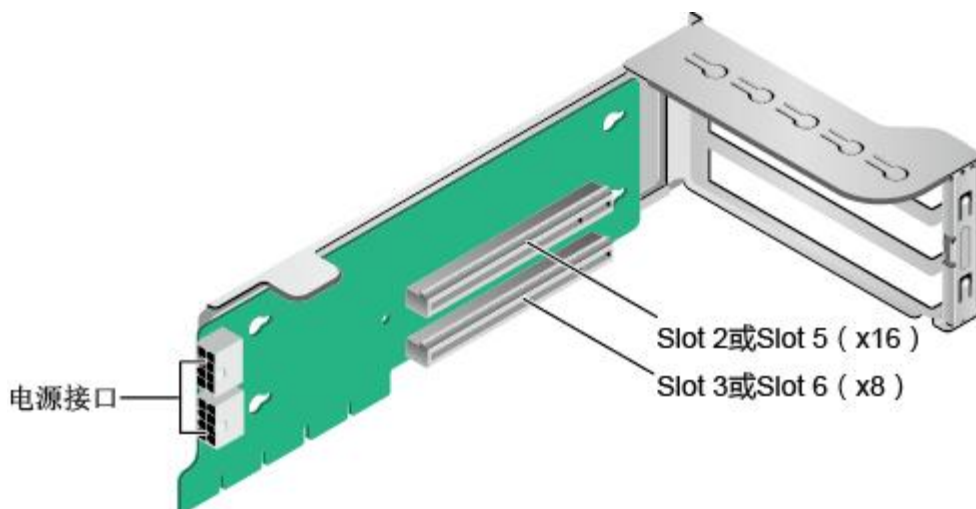
图 4-10 Riser 卡 2 (1x8+1x16)
