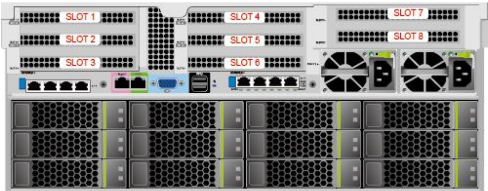
图 4-15 PCIe 插槽
