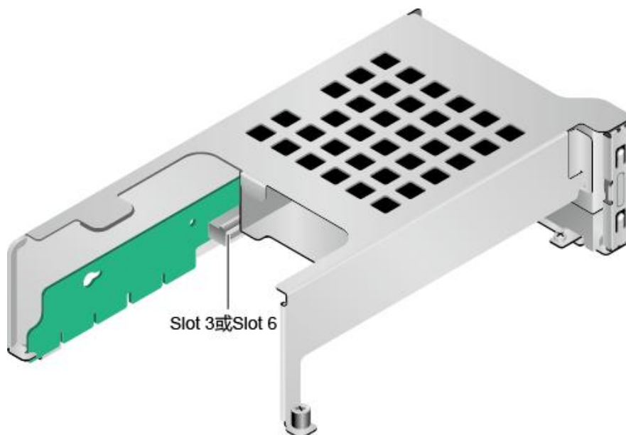
图 4-11 Riser 卡 3 (1x16)
