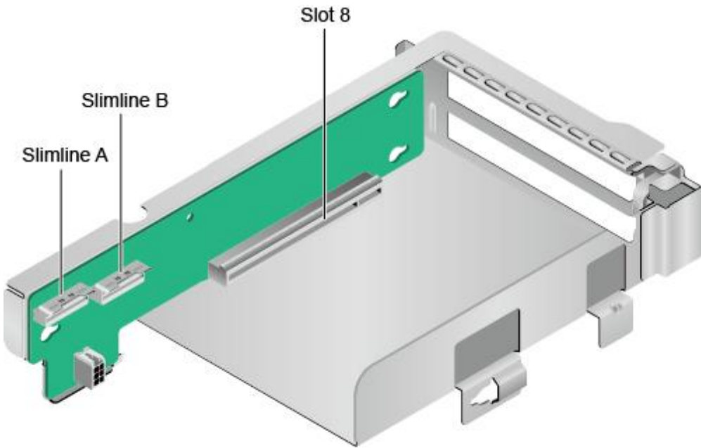
图 4-14 Riser 卡 6 (1x16)
