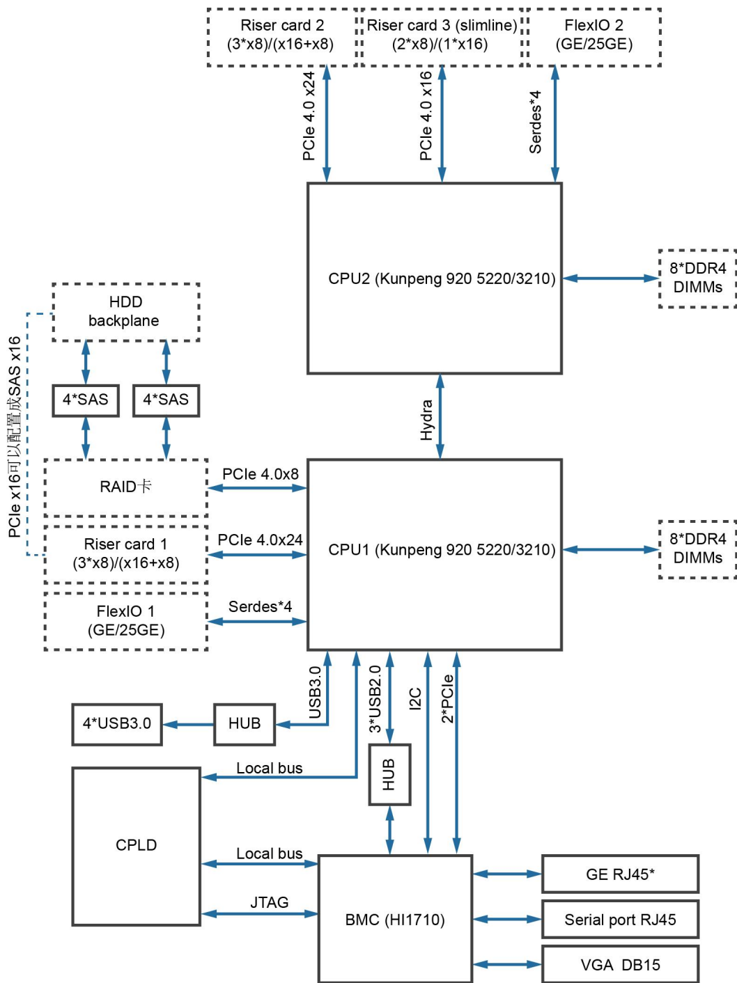
图 3-1 服务器逻辑结构
