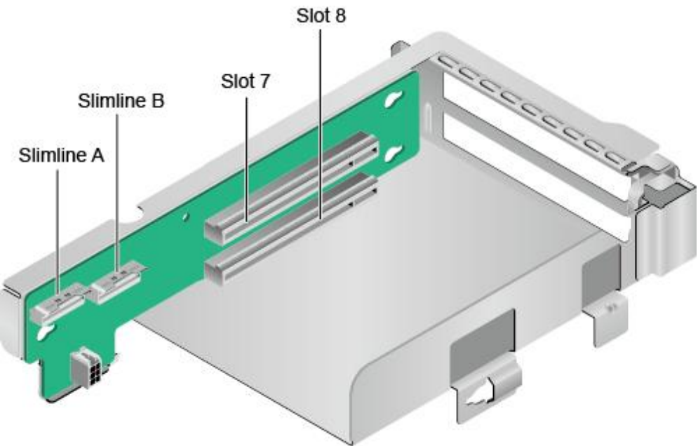
图 4-13 Riser 卡 5（2x8）
