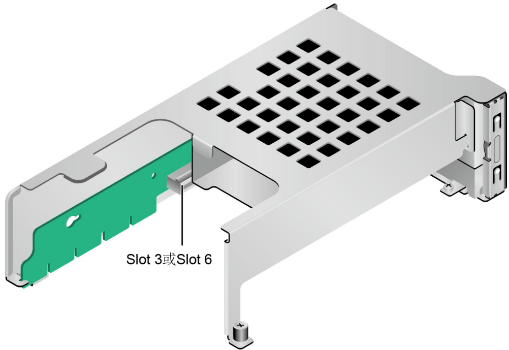
图 4-15 Riser 卡 4 (1x16)
