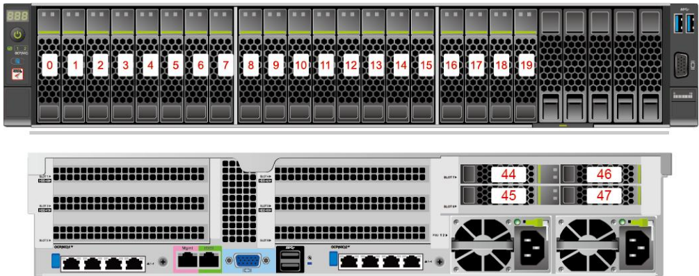
图 6-7 8x2.5 SAS/SATA+12x2.5 NVMe 硬盘配置硬盘编号
