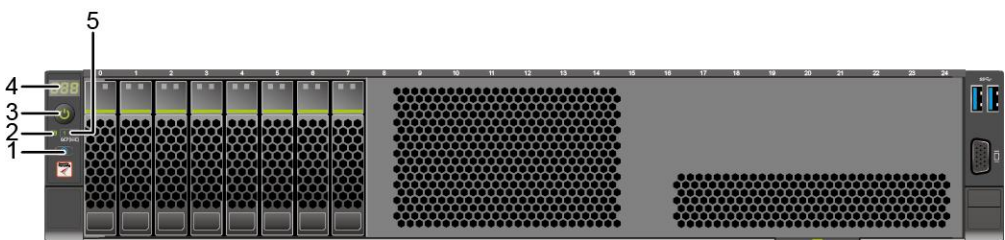
图 4-7 8x2.5 英寸硬盘配置前面板指示灯和按钮
