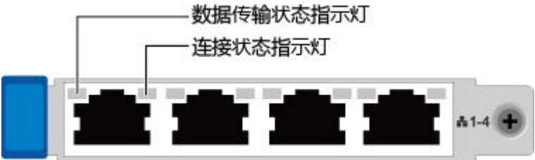
图 4-11 TM210（4*GE 电口）
