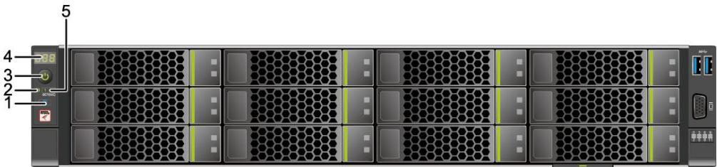
图 4-5 12x3.5 英寸硬盘配置前面板指示灯和按钮
