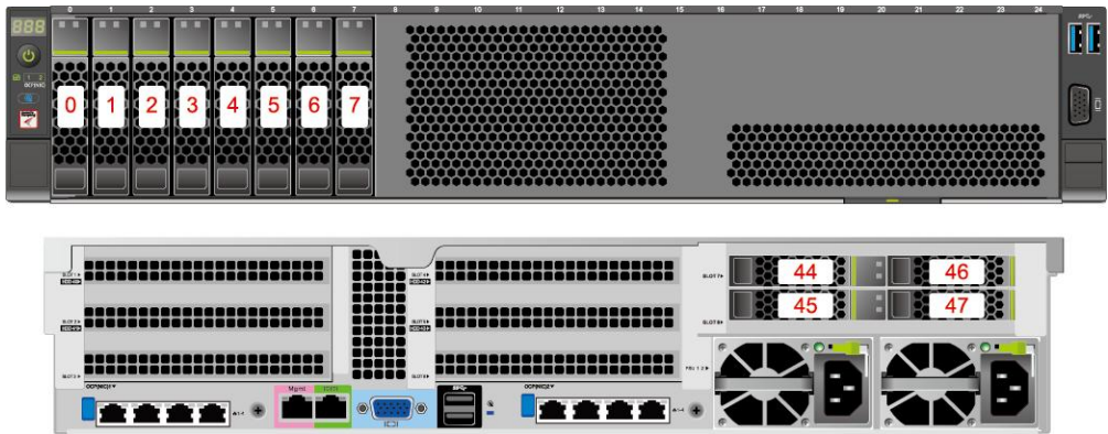
图 6-8 8x2.5 英寸硬盘配置的硬盘编号
