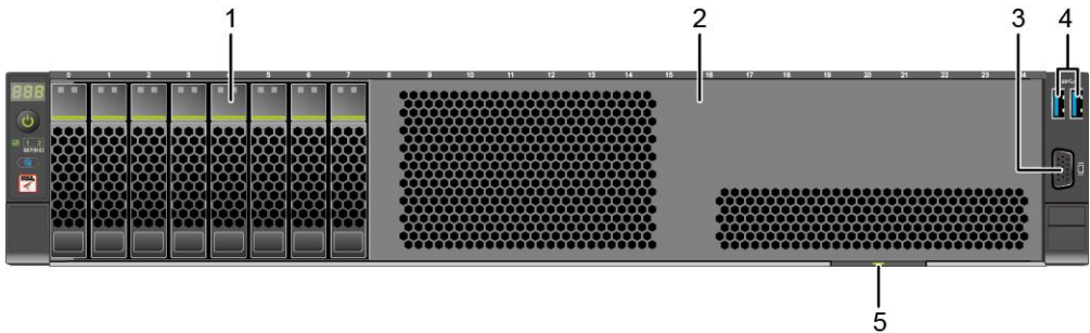
图 4-3 8x2.5 英寸硬盘配置前面板组件
