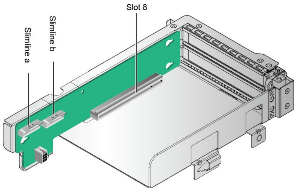
图 4-18 Riser 卡 7 (1x16)
