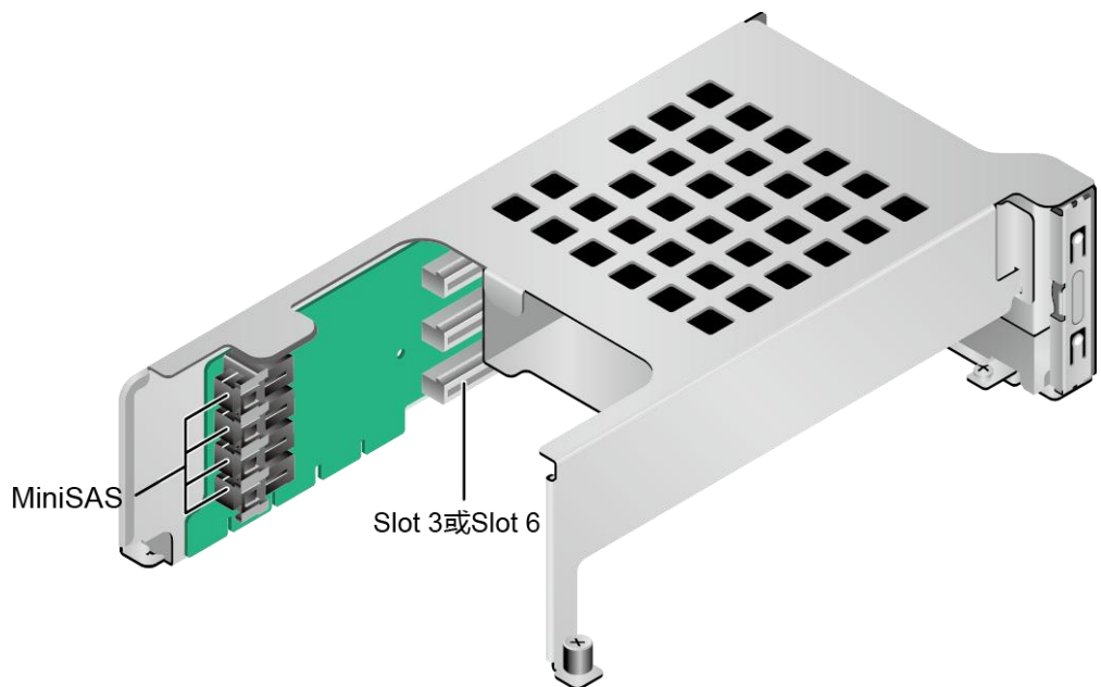
图 4-16 SAS Riser 卡 5
