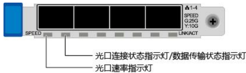
图 4-12 TM280（4*25GE 网口）
