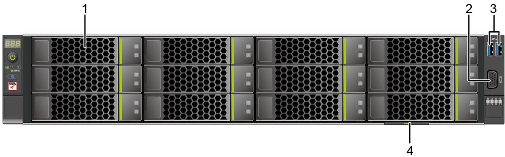
图 4-1 12x3.5 英寸硬盘配置前面板组件
