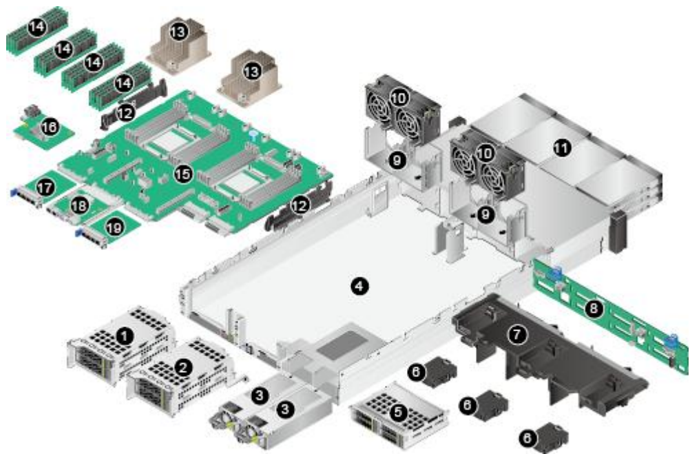
图 4-20 部件
