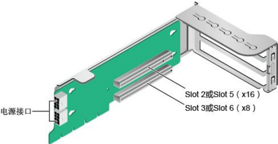
图 4-14 Riser 卡 2（1x8+1x16）
