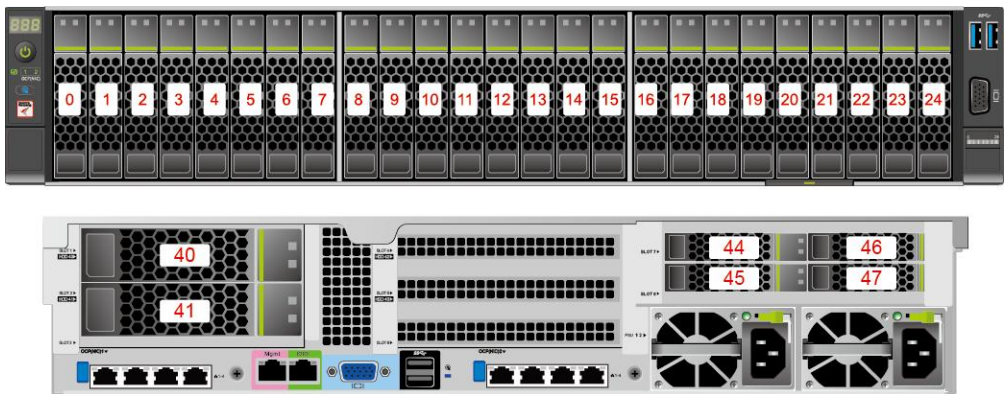
图 6-6 25x2.5 英寸硬盘 EXP 配置硬盘编号
