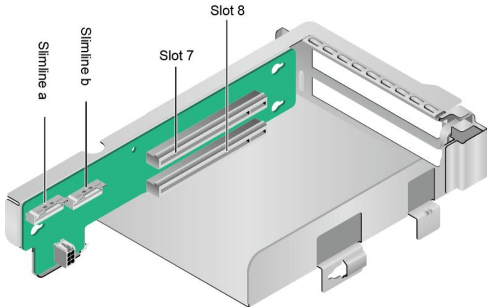
图 4-17 Riser 卡 6 (2x8)
