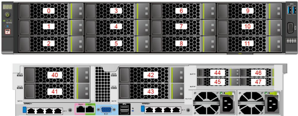
图 6-3 12x3.5 英寸硬盘 EXP 配置硬盘编号
