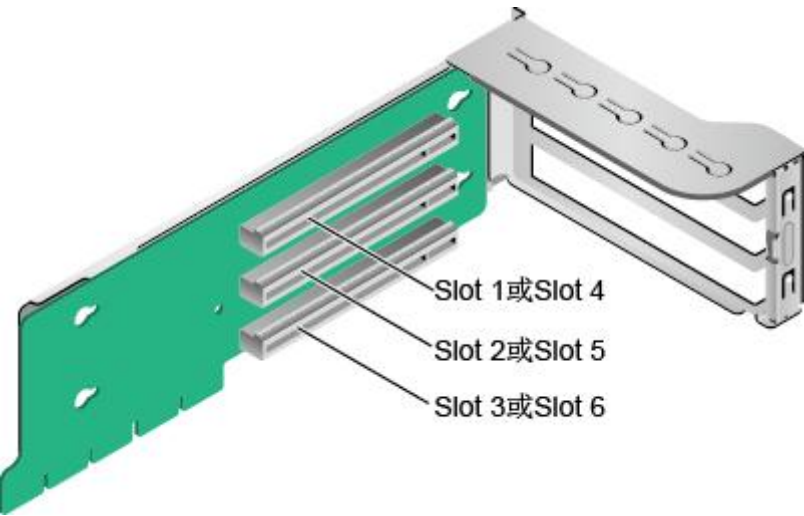
图 4-13 Riser 卡 1（3x8）
