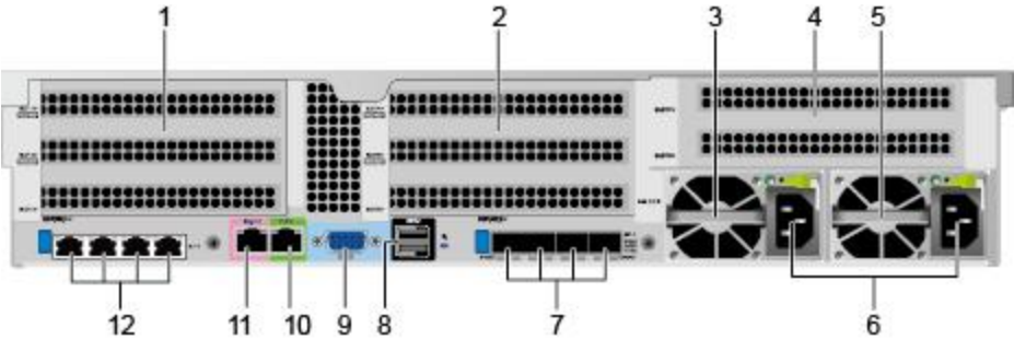
图 4-4 后面板组件
