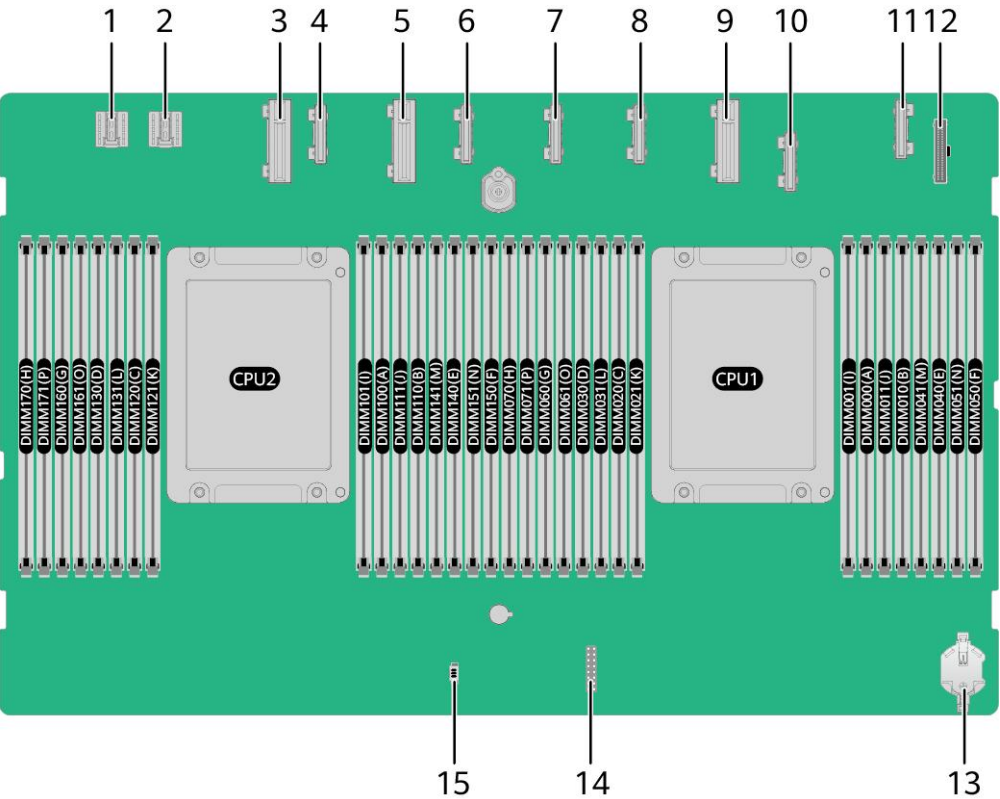
图 5-6 基础板接口
