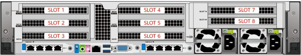
图 5-42 PCIe 插槽
