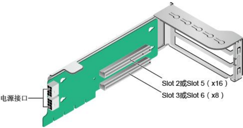
图 5-12 1x8+1x16 Riser 卡 2
