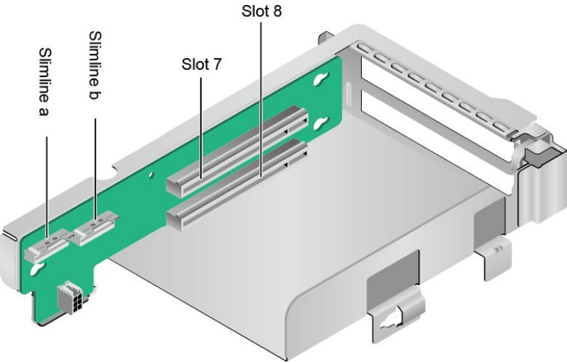
图 5-16 2x8 Riser 卡 6
