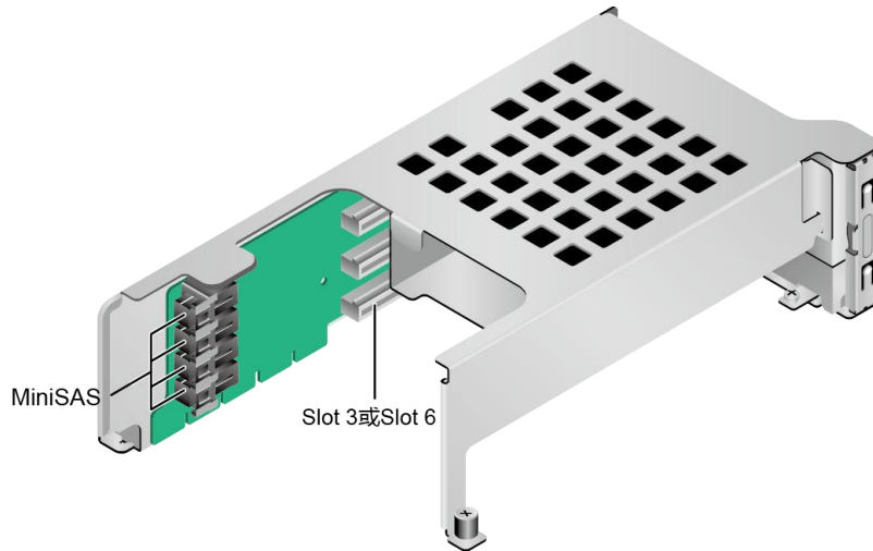
图 5-14 2x2.5 背板 SAS Riser 卡 4
