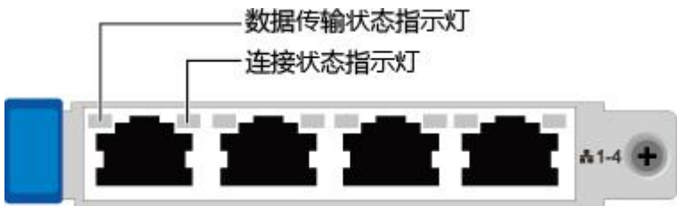
图 5-5 TM210（4*GE 电口）
