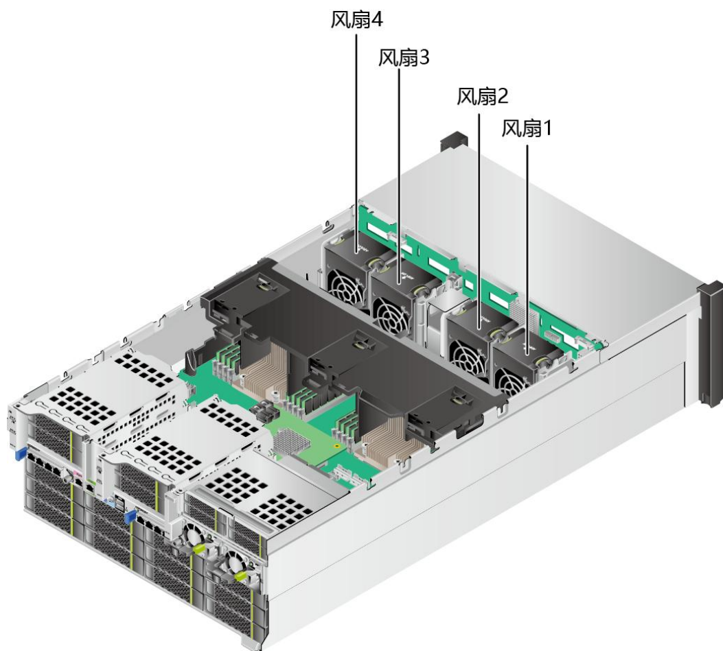
图 5-19 风扇位置图
