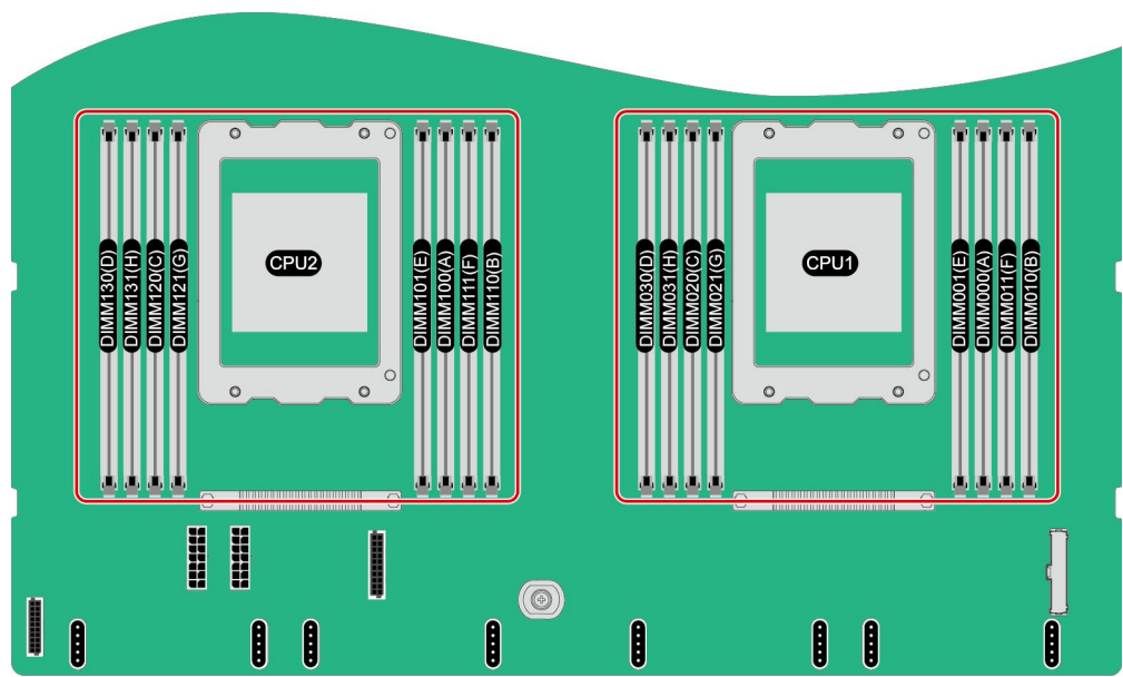
图 7-1 内存槽位编号
