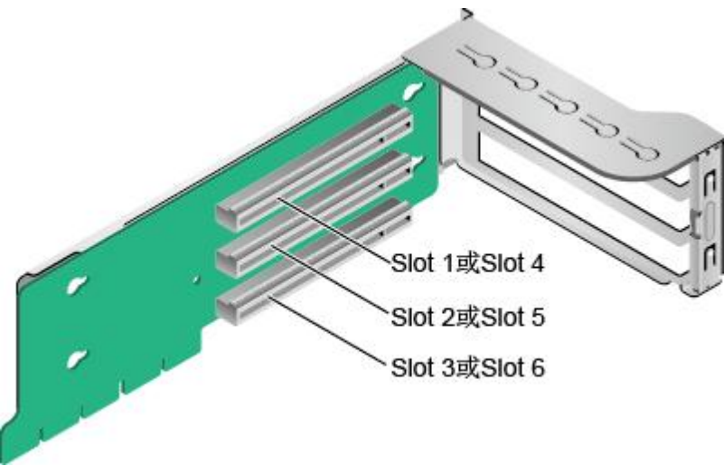
图 5-11 3x8 Riser 卡 1
