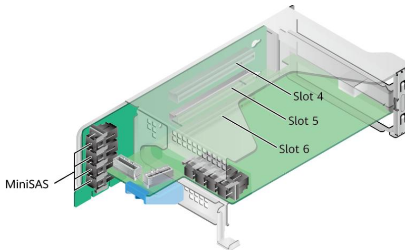
图 5-15 IOB 卡 SAS Riser 卡 5
