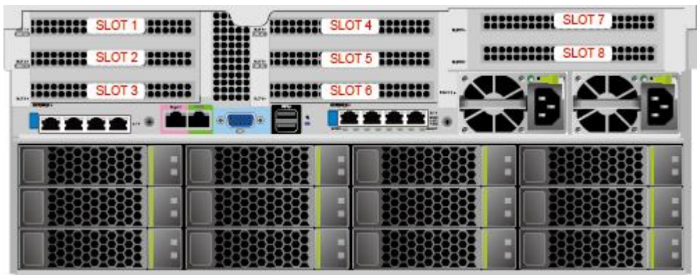
图 5-18 PCIe 插槽
