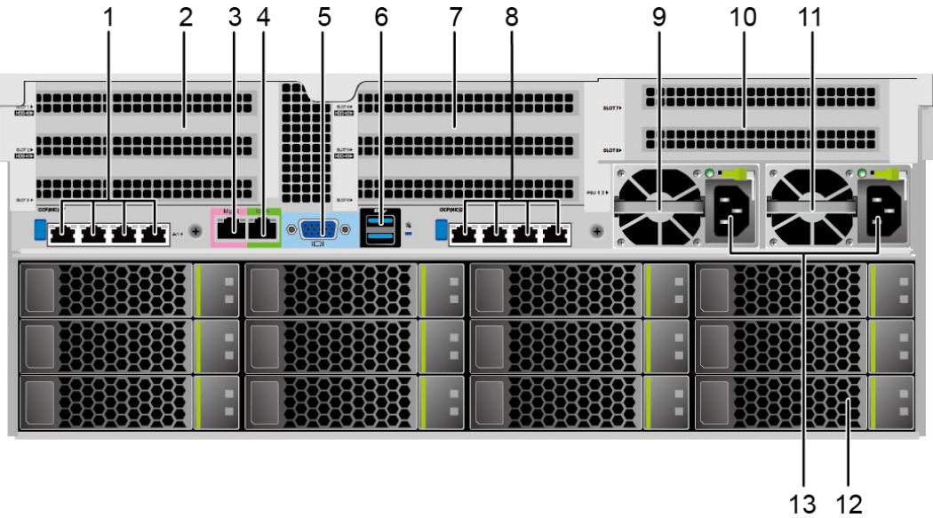
图 5-3 后面板组件
