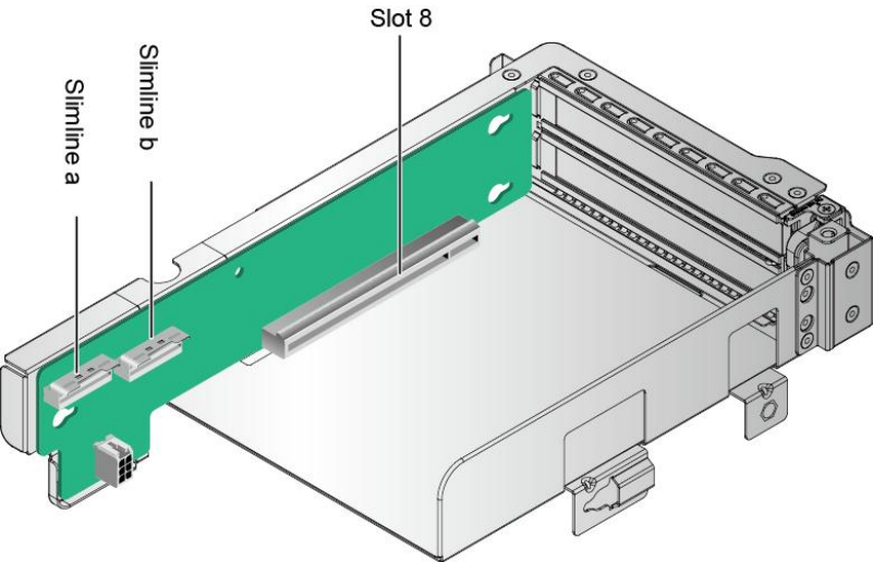
图 5-17 1x16 Riser 卡 7
