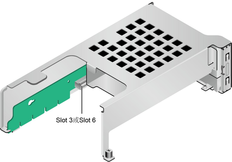
图 5-13 1x16 Riser 卡 3
