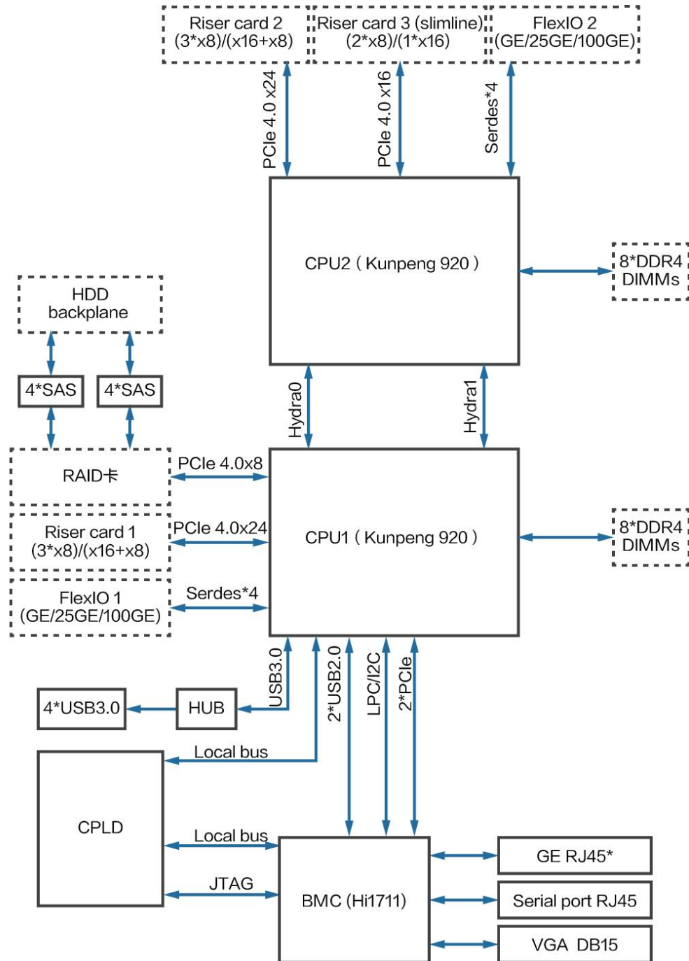
图 4-1 服务器逻辑结构
