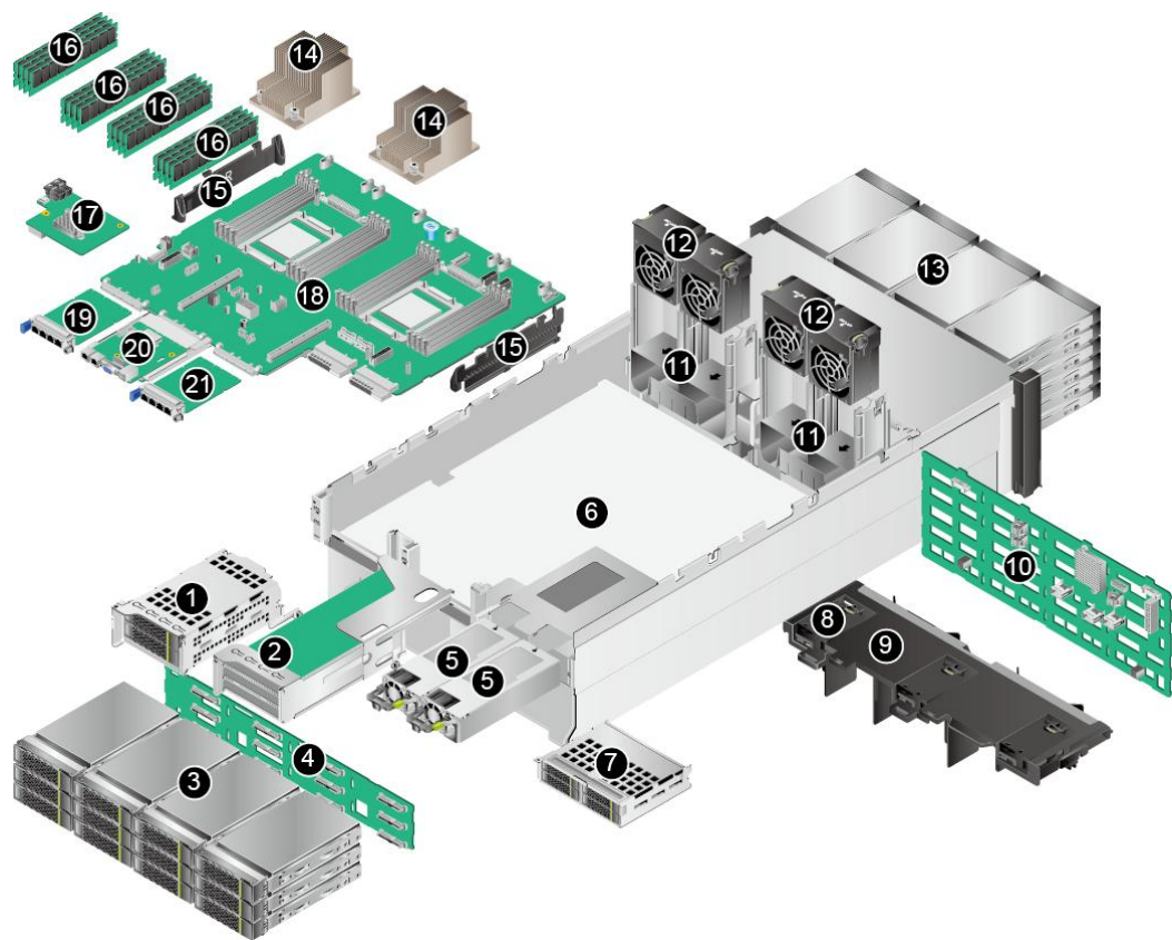
图 3-1 部件
