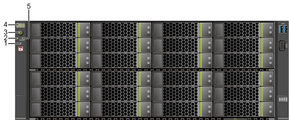
图 5-2 前面板指示灯和按钮
